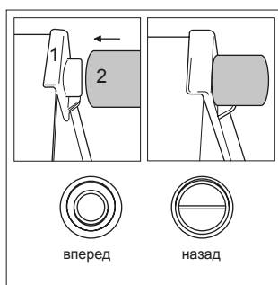
Рис. 2. Установка ограничительных упоров
